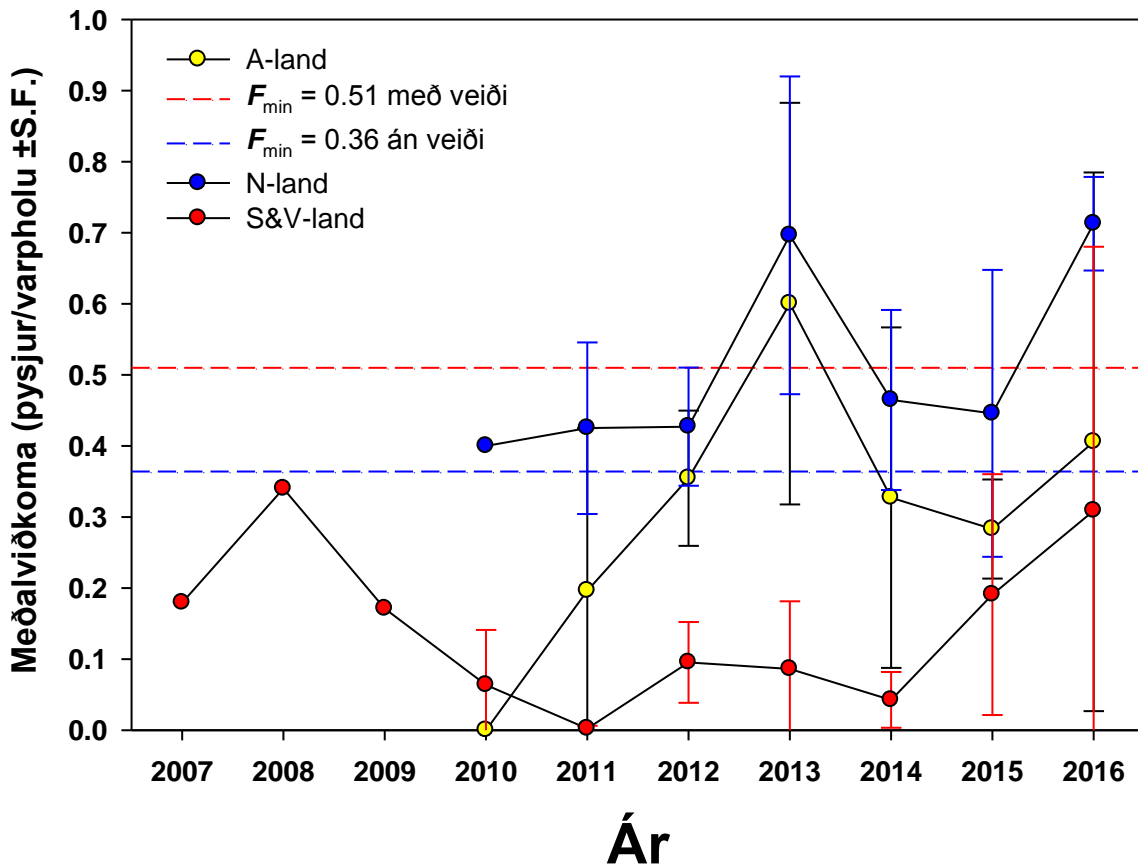
2. Mynd. Meðalviðkoma ( \pm staðalfrávik) eftir landsvæðum 2007-2016. Svæðaskipting er við Gölt, Font og Eystra Horn. Til viðmiðunar er sýnd útreiknuð lágmarksviðkoma ( F_{min} ) með og án veiða þannig að stofnvöxtur sé engin, viðkoma þarf að vera yfir F_{min} til að stofnvöxtur eigi sér stað. Litlar veiðar eru utan norðursvæðis.
